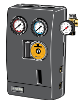
NIBE Aurinkopumppuasema SPS10 *Tuotenro 057027 (1 kpl)
