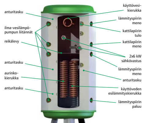
Oilon-hybridivaraaja
